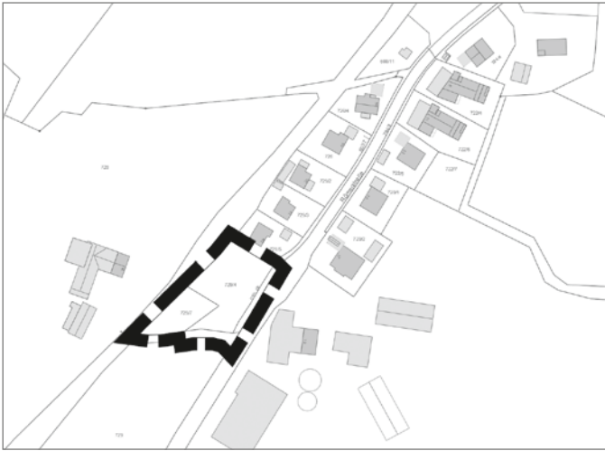
Abbildung 2: Lageplan der 18. Änderung im Bereich Römerstraße – Ermengerst, unmaßstäblich
